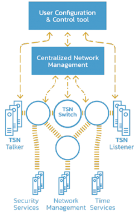
TSN网络拓扑
